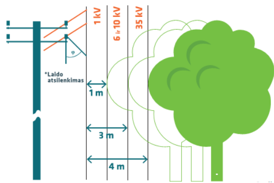
Laido atsilenkimas – tai galimas laido svyravimo atstumas, pavyzdžiui, pučiant stipriam vėjui.
